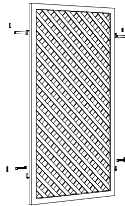
㊦ ラチス H:1,855 W:1,025 t:45 白塗装
