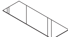
(b)-2 オープンケース棚ガラス W:1189 D:389 t:6 クリアーガラス
