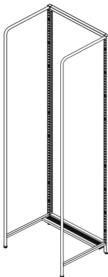
(a) タワー本体 H : 2100 W : 630 D : 500 スチールフレーム：粉体塗装仕上
