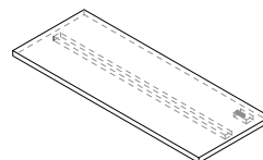
(b)-2 棚板(大) W : 1200 D : 450 t : 25 天面：シナ合板クリア塗装仕上 見付：木口テープ(ストライプウッド) 照明：ラインLED N900 内蔵 消費電力：10.8W
