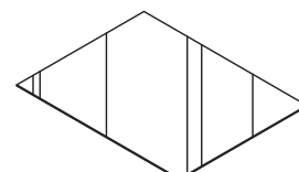
(c)-1 オープンケースワイドトップガラス W:1029 D:796 t:6 クリアーガラス
