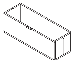
(b)-5 オープンケース用ストックBOX H:400 W:1150 D:395 天面：シナ合板クリア塗装仕上 見付：木口テープ(ストライプウッド)
